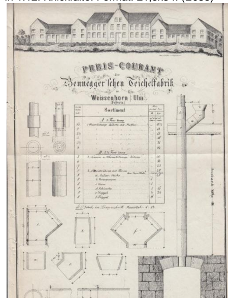
Los 957 Ausruf: 30 € Weissenhorn/Ulm, ca. 1880: Benneger'sche Teichelfabrik, Preis-Courant Einseitig. Abb. der Firma. Preislistung; Quer- und Längsschnitte einiger Produkte. Formate in 1:12. Knickfalte. Format: 21,5x34. (E033)
